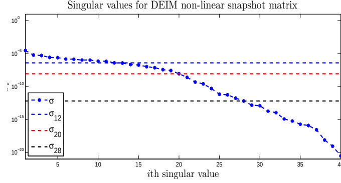
FIG. 5.4. Singular values of the POD-DEIM snapshot matrix.
